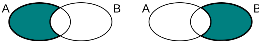
Figura 5.23: Diferencia. El resultado de A menos B es solo lo que está en A y no en B.
