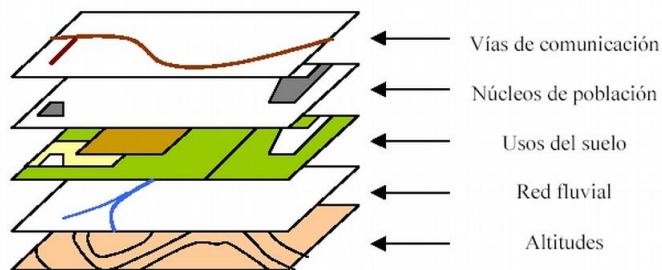
Figura 1.3: Esquema de capas de información en un SIG. Fuente: Wikipedia
