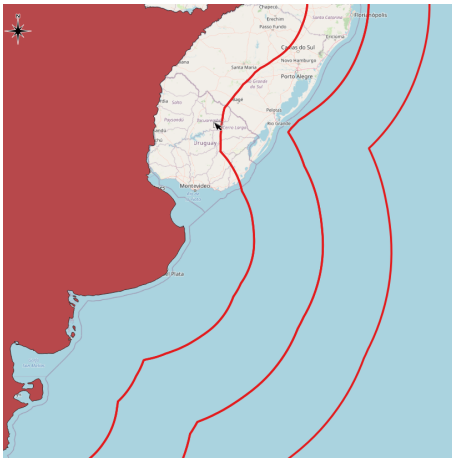
Figura 5.19: Buffer de 300km segmentado en 3 sectores.
