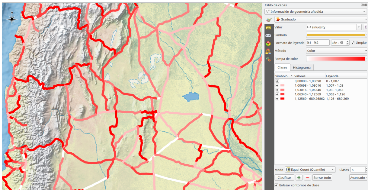
Figura 5.36: Índice de sinuosidad. Colores rojizos fuertes indican mayor sinuosidad.
