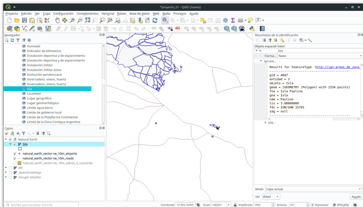
Figura 2.19: Capa de Islas del IGN Ar.
