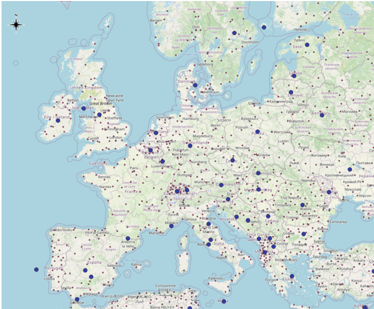
Figura 5.33: Coordenadas medias. Los puntos violetas pequeños pertenecen a la capa de ciudades, y los azules más grandes a sus respectivos centros de gravedad calculados por grupos donde el atributo es el nombre del país al que pertenecen.
