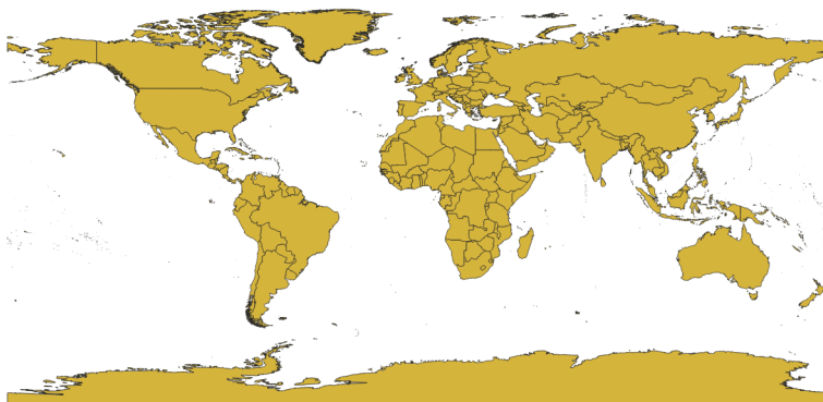
Figura 2.5: Límites Administrativos con resolución de 10m.
