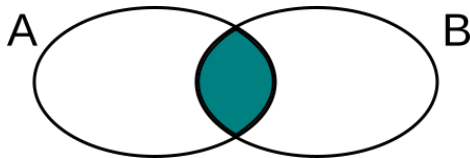
Figura 5.20: Intersección. El resultado son los elementos comunes entre las dos geometrías.
