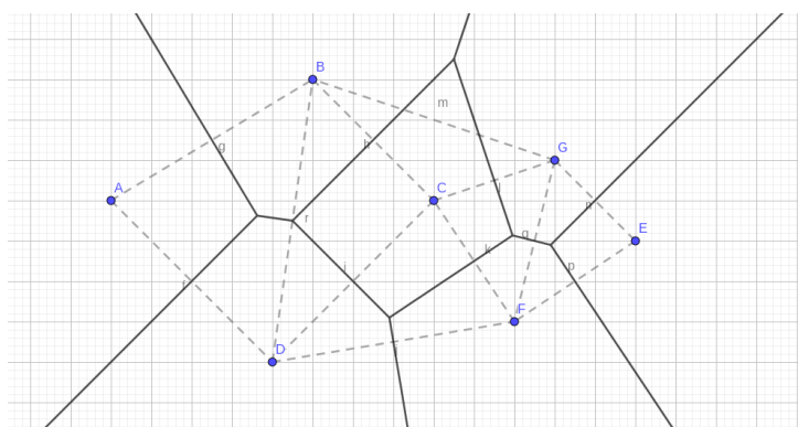
Figura 5.27: Polígonos de Voronoi. Los segmentos en color negro conforman los lados de los polígonos, y son las mediatrices de los segmentos que unen pares de puntos vecinos. Gráfica realizada con GeoGebra.
