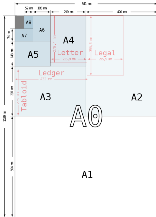
Figura 4.1: Familia de formatos de hoja serie A. Se superponen algunas hojas de otros formatos tradicionales a modo de comparativa. Fuente Wikipedia.
